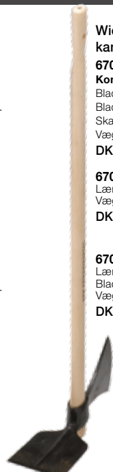
Wiederhofhakke oval 670175 Komplet med skaft Bladlængde: 45 cm. Bladbredde: 16/12,5/9 cm. Skaftlængde: 105 cm. Vægt: 2,5 kg. DKK 270,00 (337,50)
