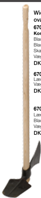
Ulmer plantehakke 670190 Længde: 135 cm. Bladbredde: 12 cm. Bladlængde: 18 cm. Vægt: 1,35 kg. DKK 199,00 (248,75)
